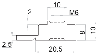
ZDC Nut - M6
