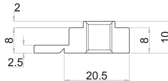
ZDC Nut - M8
